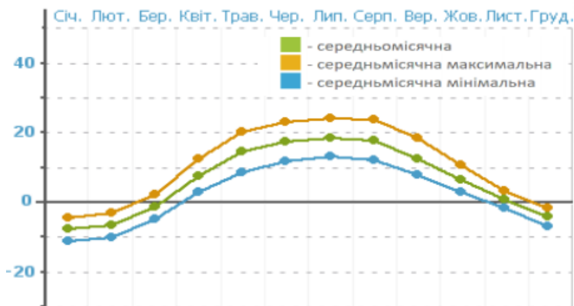
Рисунок 2.1 Середня місячна і річна температура повітря ( ^{\circ}\text{C} )
